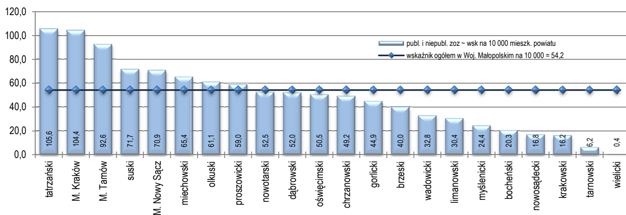
Rysunek 13. Wskaźniki liczby łóżek w jednostkach opieki stacjonarnej (publicznych i niepublicznych) na 10 000 mieszkańców subregionu w 2011 r.
